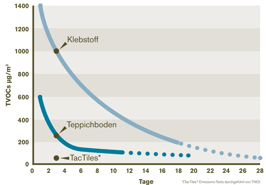
Typische Emissionsabklingkurven mit Schwellenwerten für Klebstoff und Teppichböden
